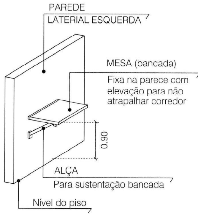
PERSPECTIVA FIXAÇÃO NA PAREDE 1 SEM ESCALA
