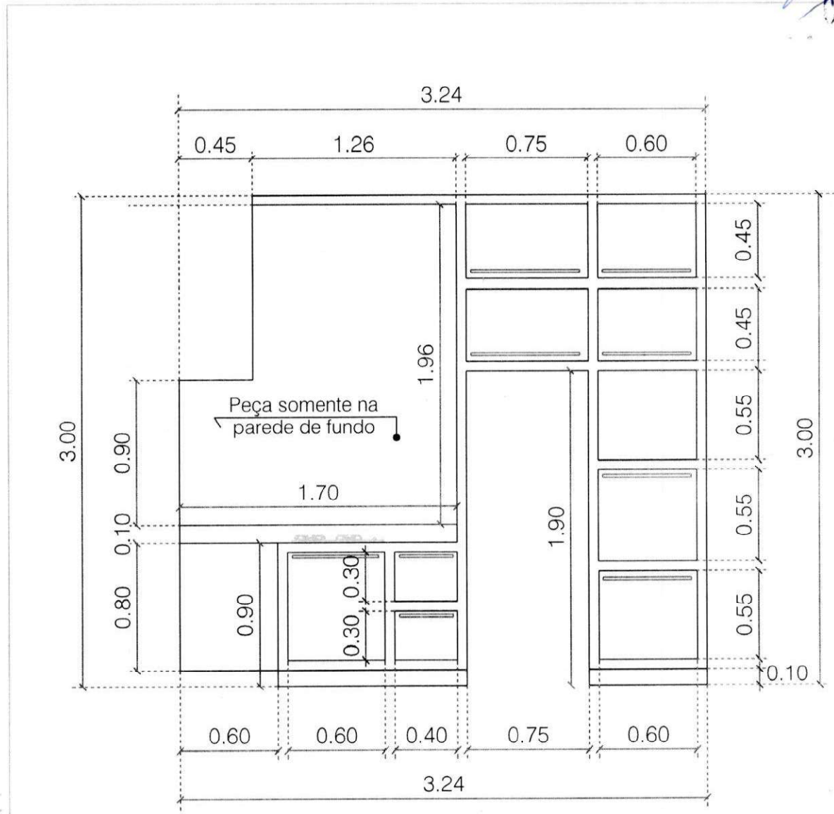
ELEVAÇÃO FRONTAL PAREDE LATERAL DIREITA
